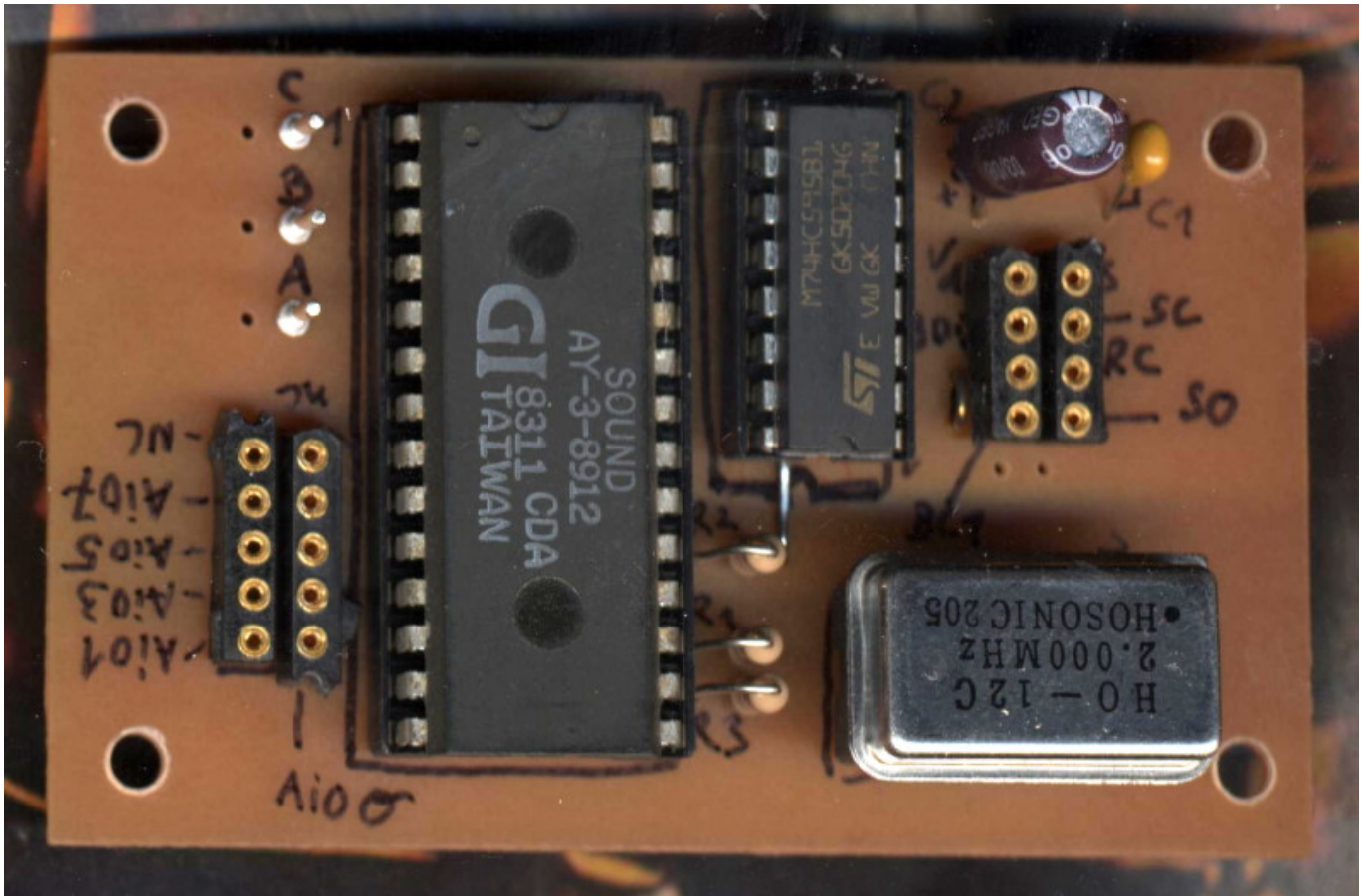
[MIDIBox AY V1 - AY 3 8912 Module]
