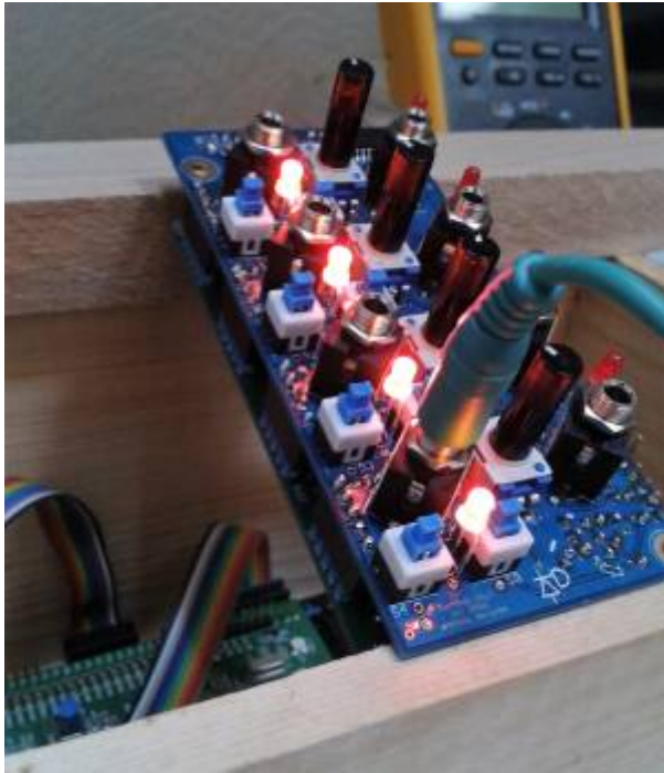
PAD_4*4 ENC_4*4
